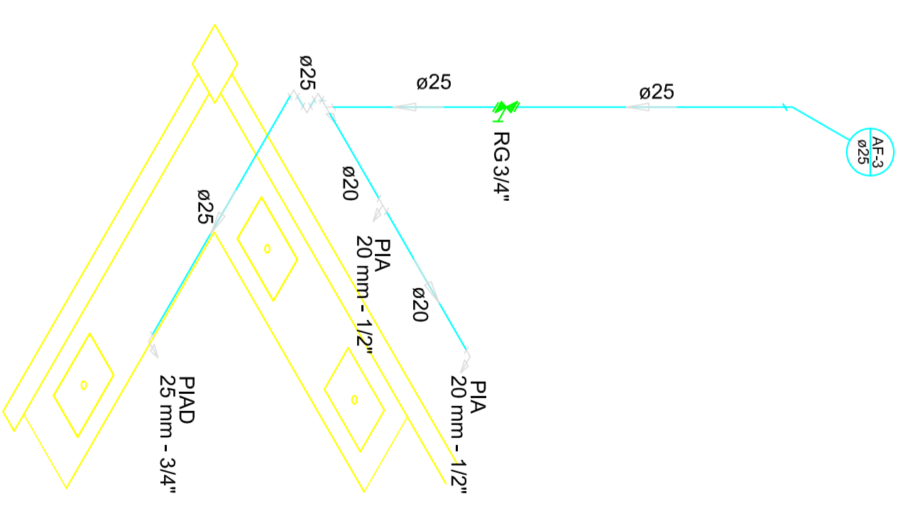
ÁREA DE LIMPEZA DE LOUÇAS Detalhe H3
