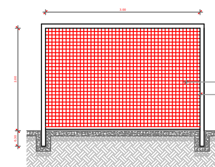
BALISA FUTEBOL VISTA FRONTAL
